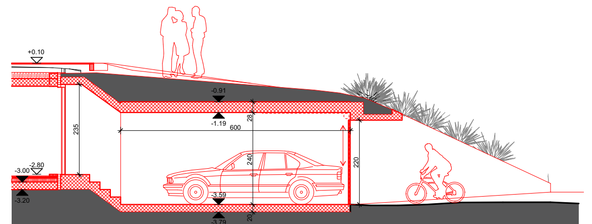
Coupe H-H
