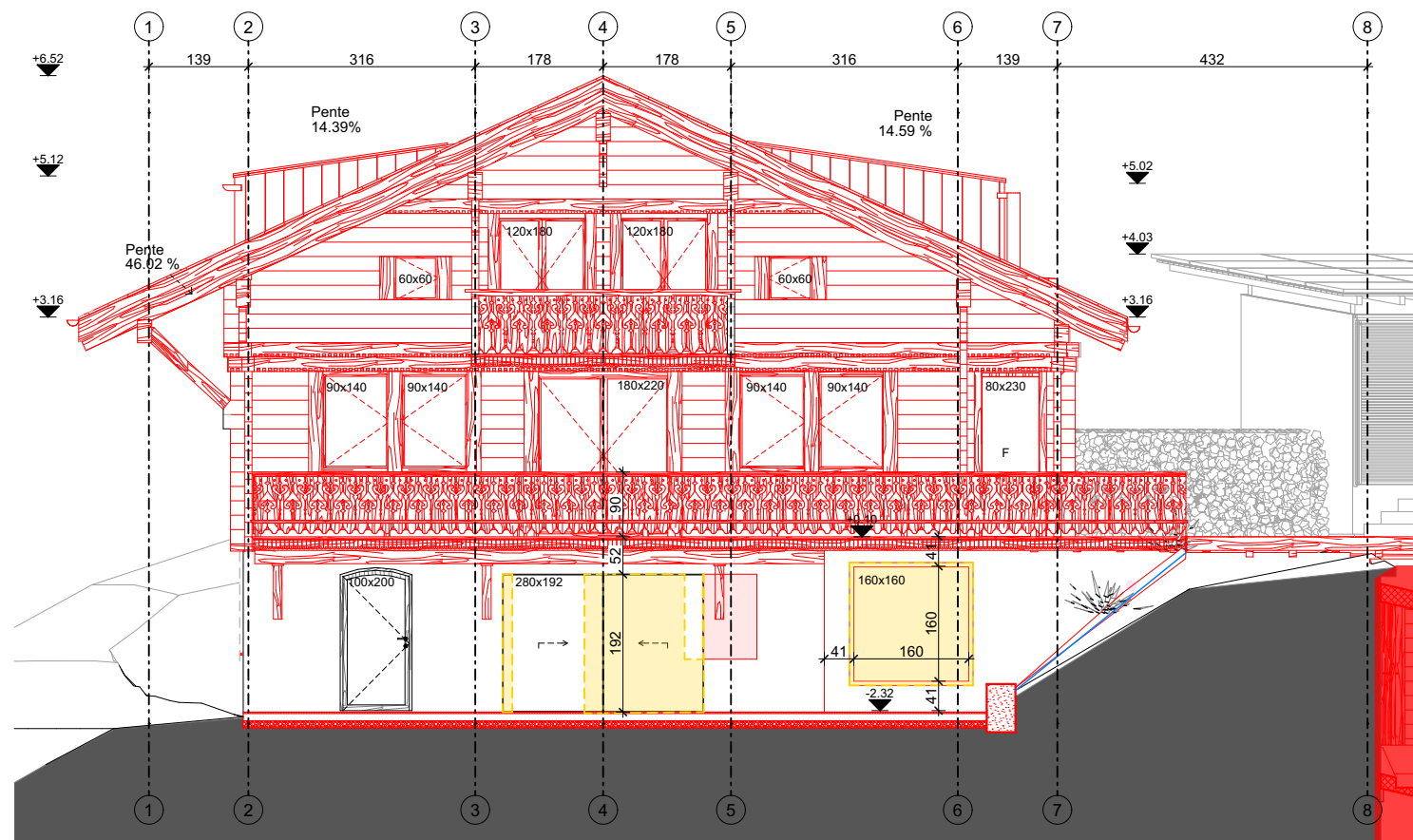
Façade S-O
