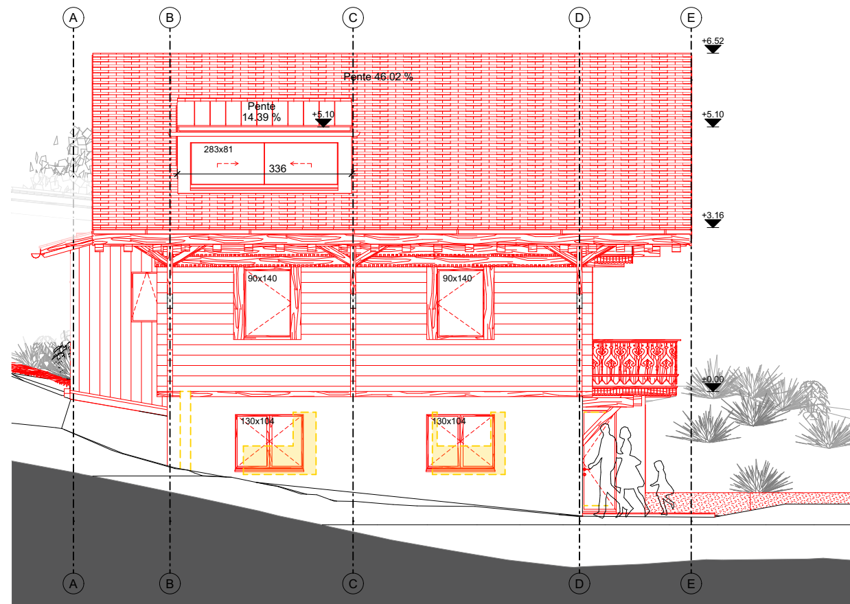
Façade N-O
