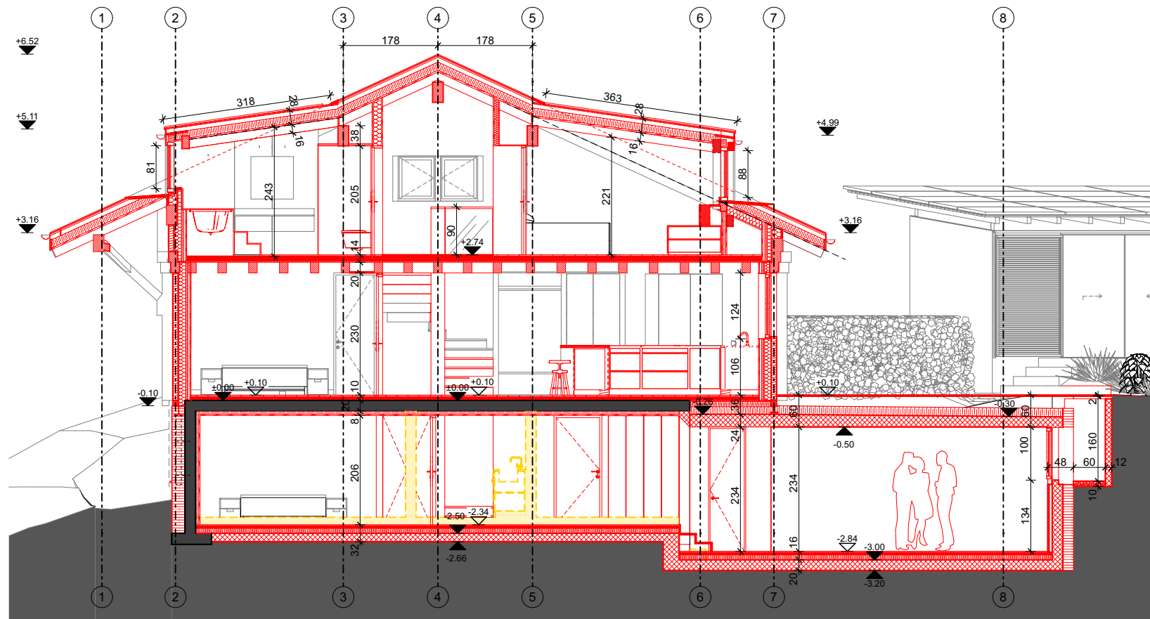
Coupe BB
