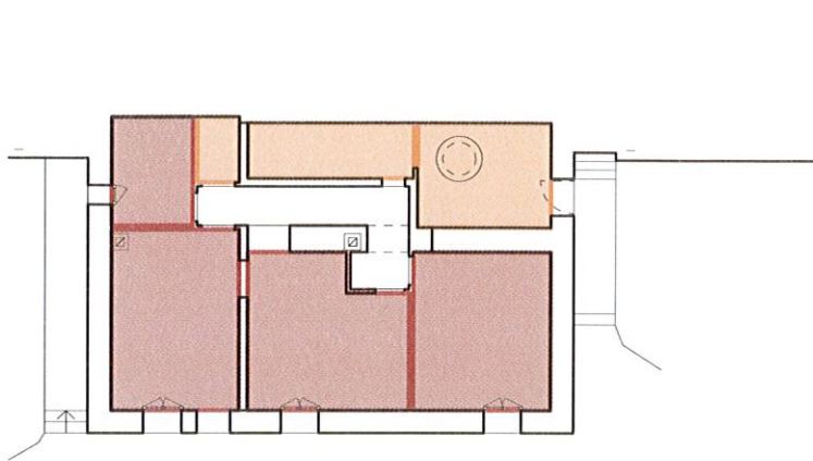
Surfaces de plancher existantes
