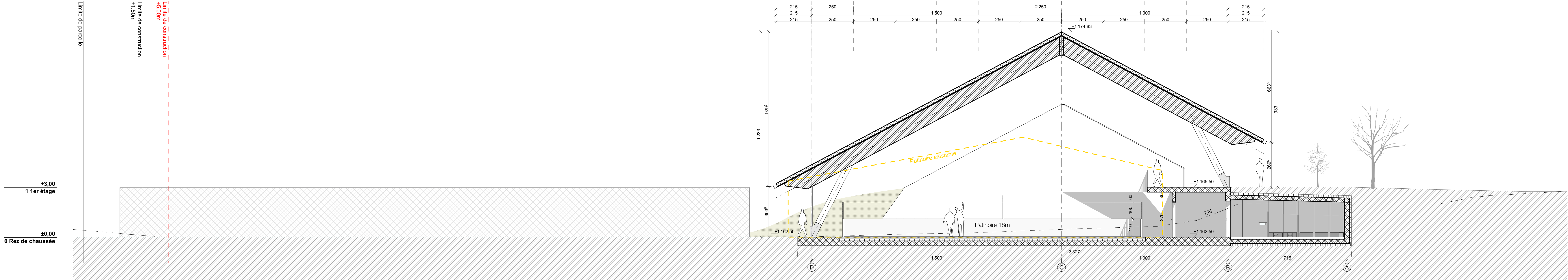
Coupe A-A - Ech 1:100
