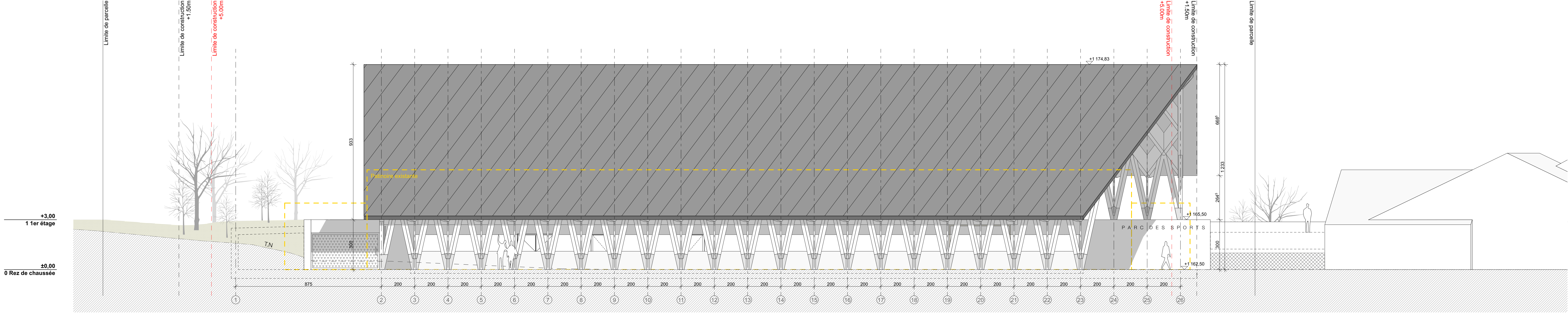
Elévation Nord-Est - Ech 1:100
