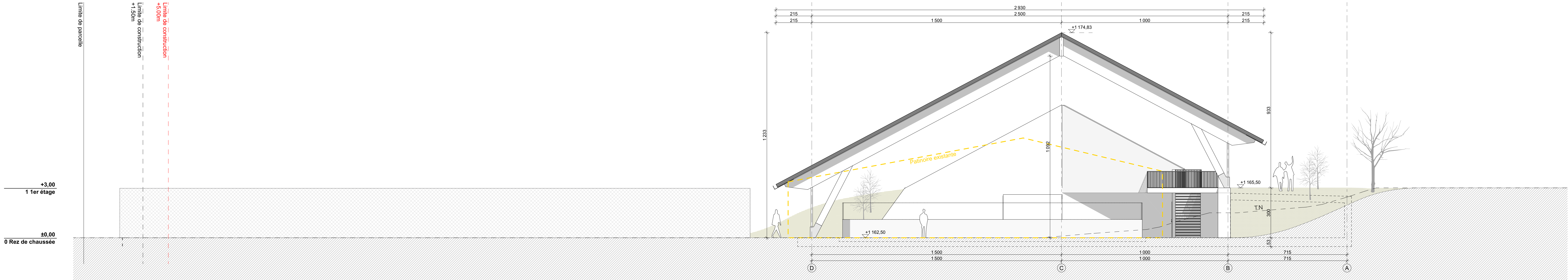
Elévation Nord-Ouest - Ech 1:100
