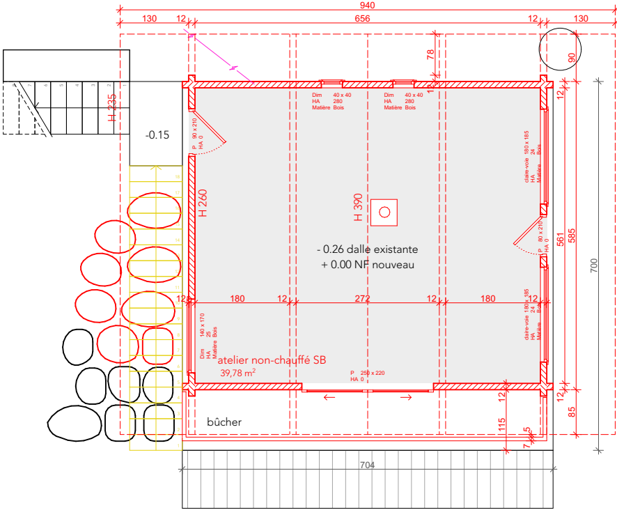
Plan rez-de-chaussée | 1:100
