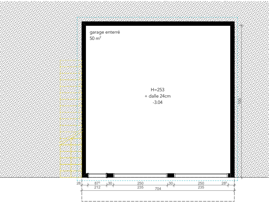
Plan sous-sol | 1: 100
