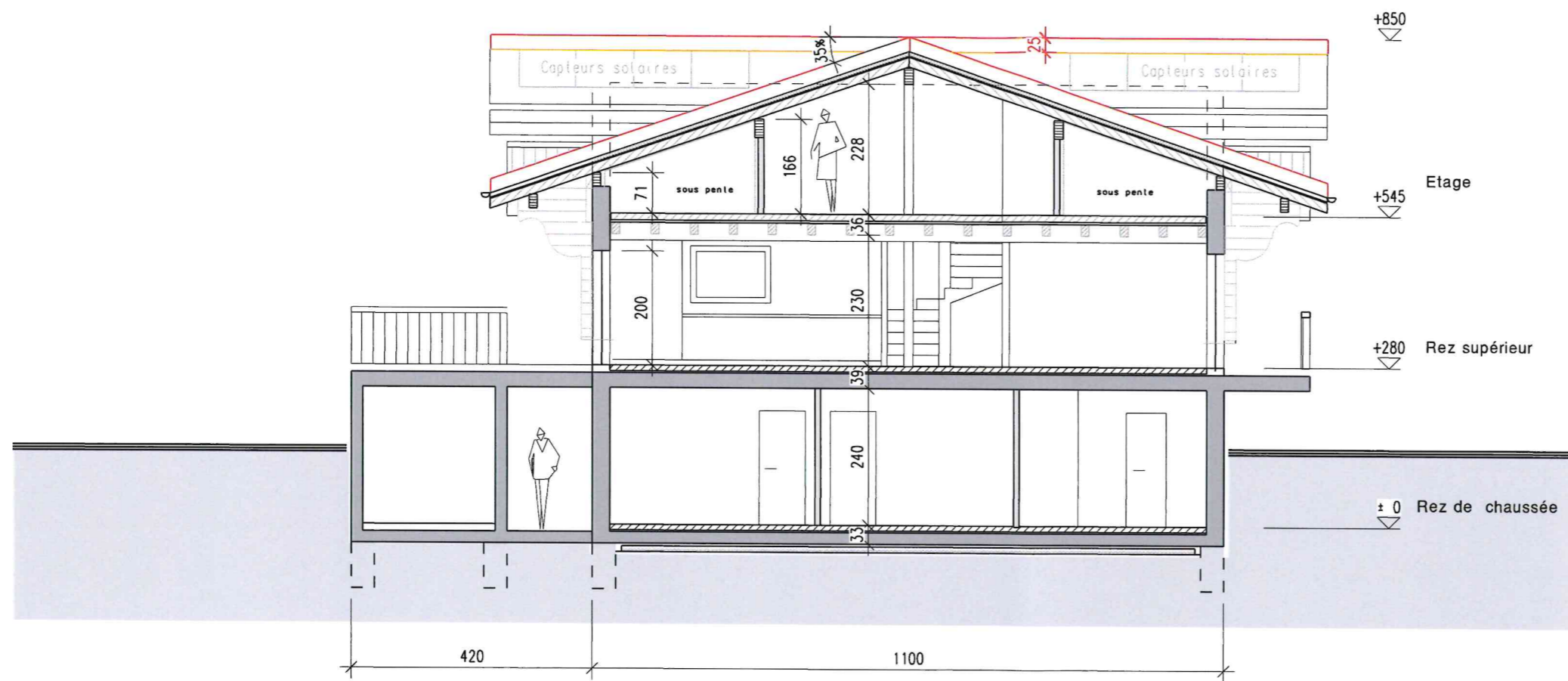
Coupe A - A
