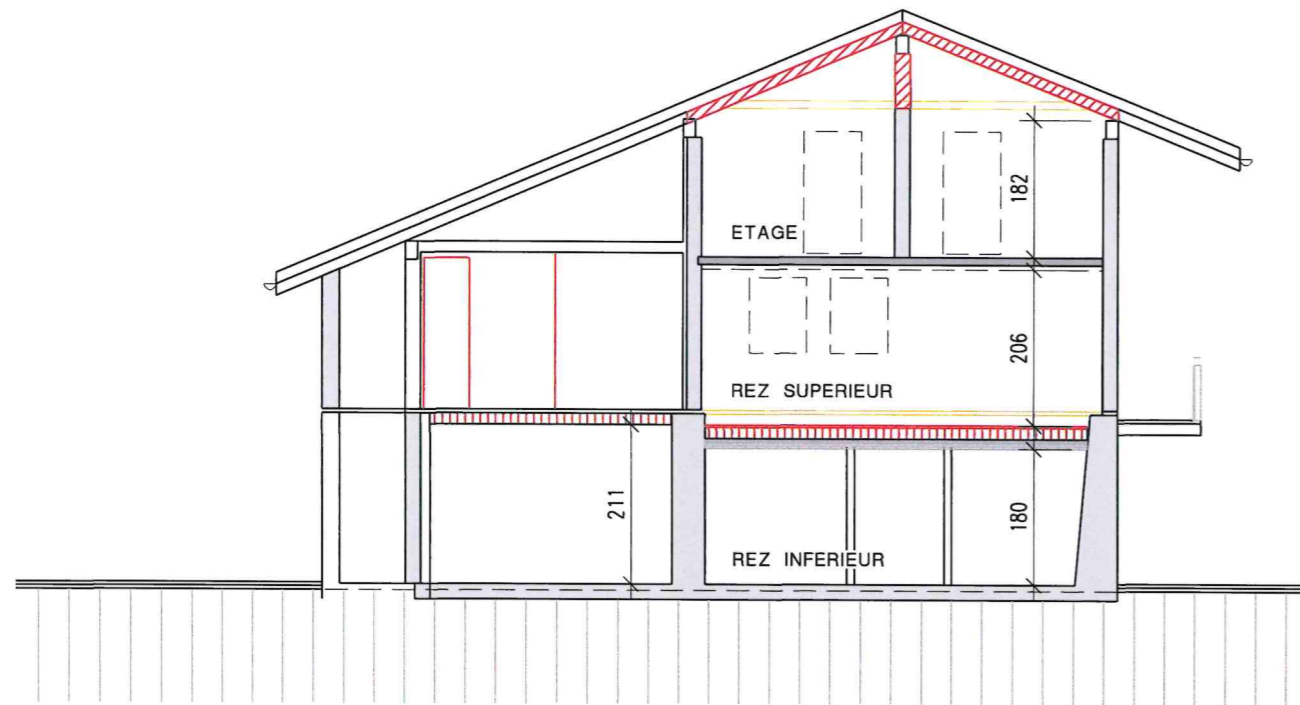
COUPE A - A
