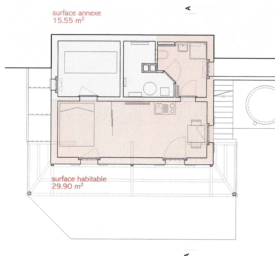
Etat 2024 Rez-Inférieur - 1:100
