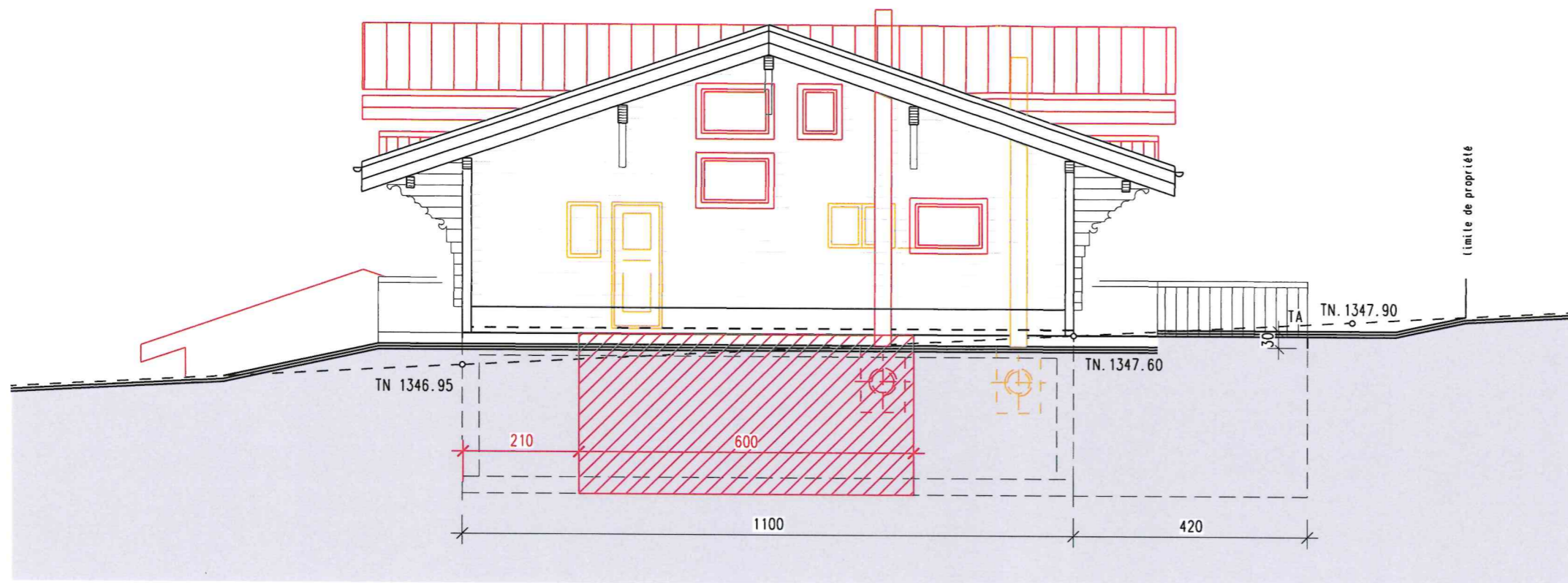
Façade NORD
