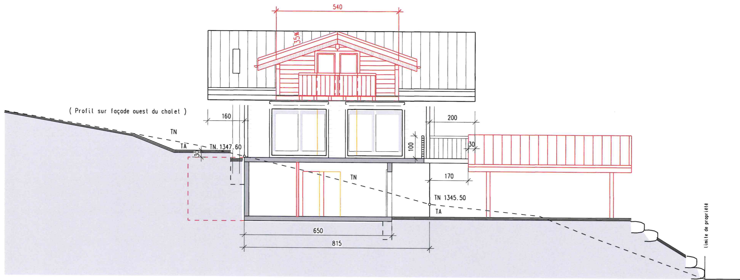
Coupe B -B Façade OUEST du chalet
