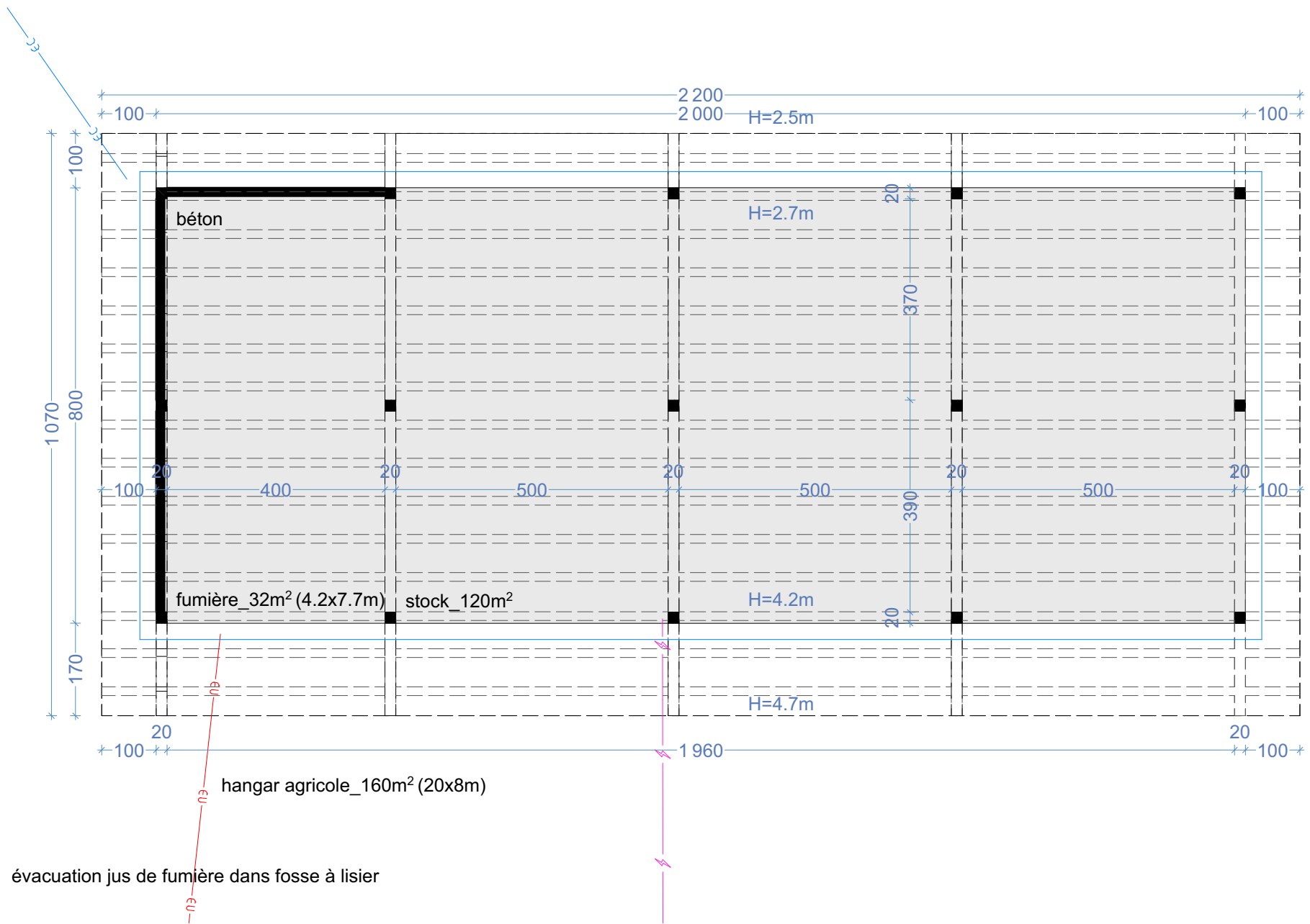
Plan rez-de-chaussée | 1:100
