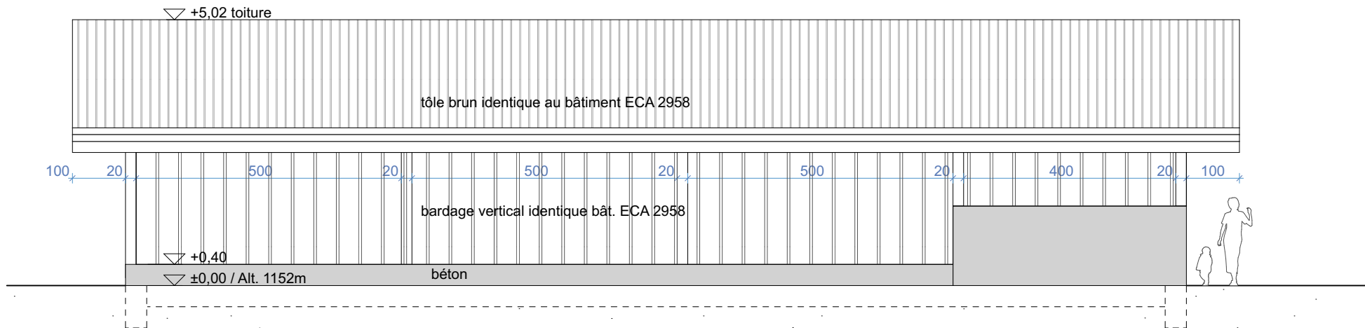
Façade NORD | 1:100
