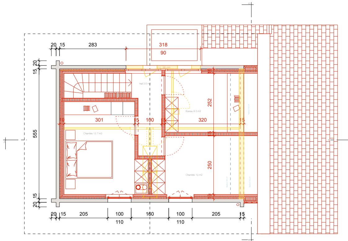
Plan de l'étage 1:100
