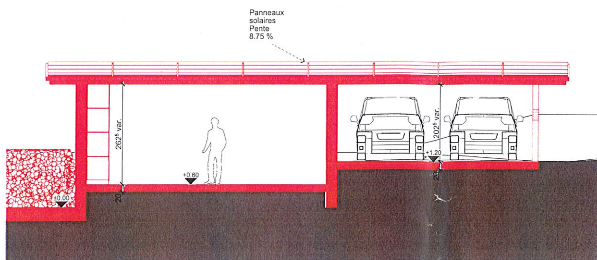
COUPE D
