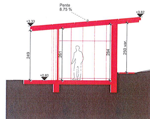
Coupe E
